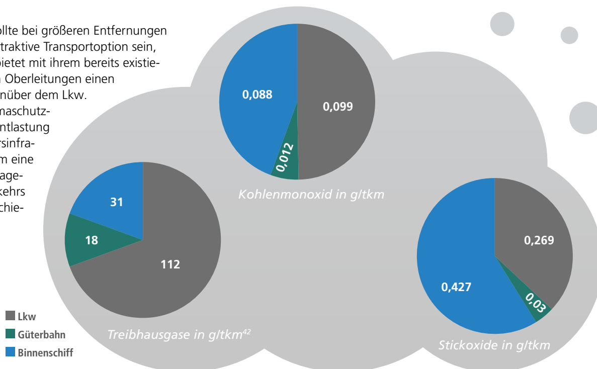
Grafik 10: Vergleich der durchschnittlichen Emissionen einzelner Verkehrsmittel im Güterverkehr (Bezugsjahr 2018)
